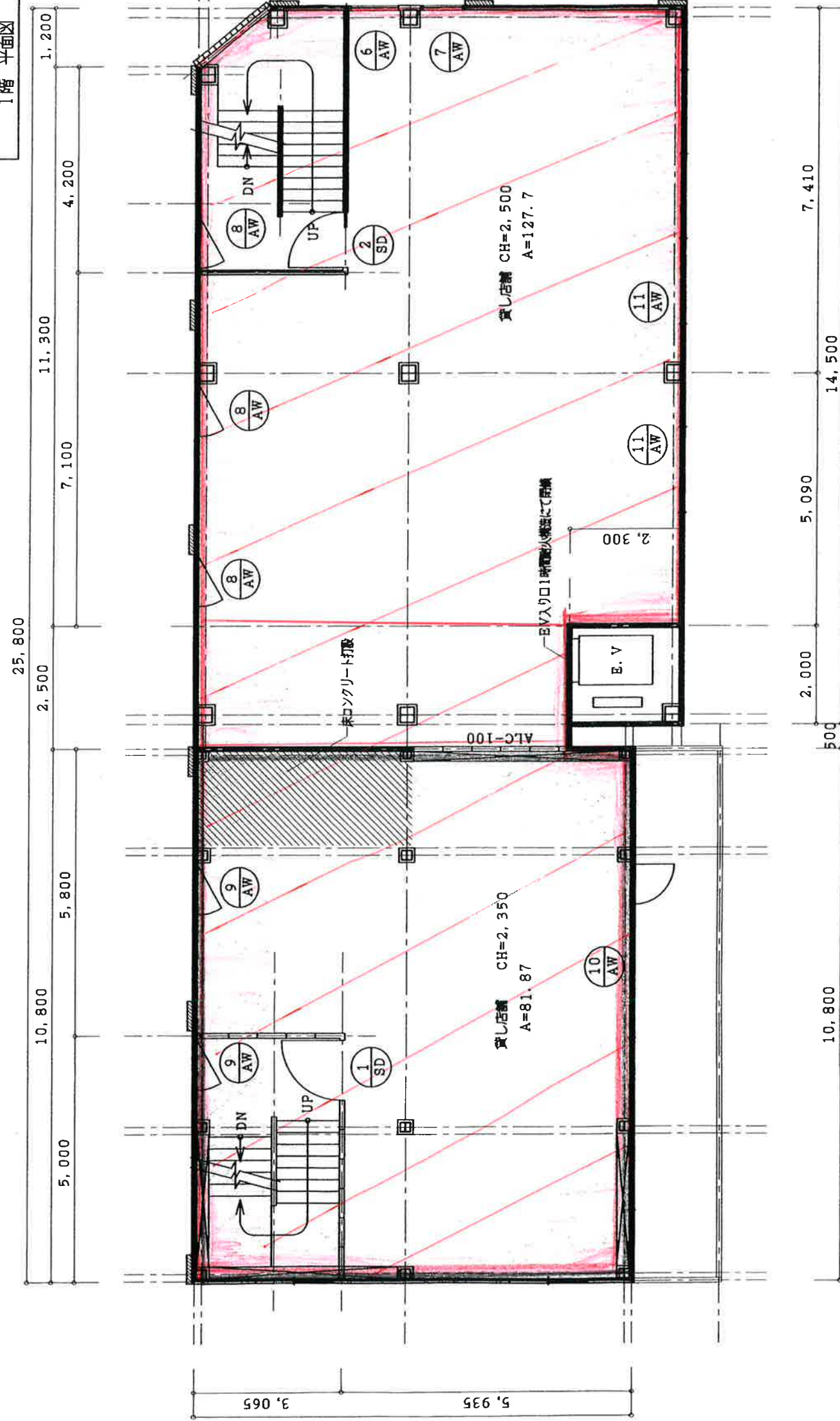
2階 平面図
