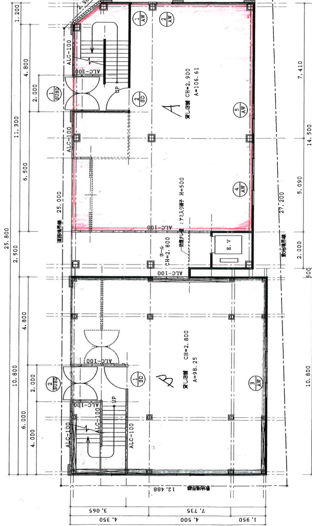
1階 平面図
